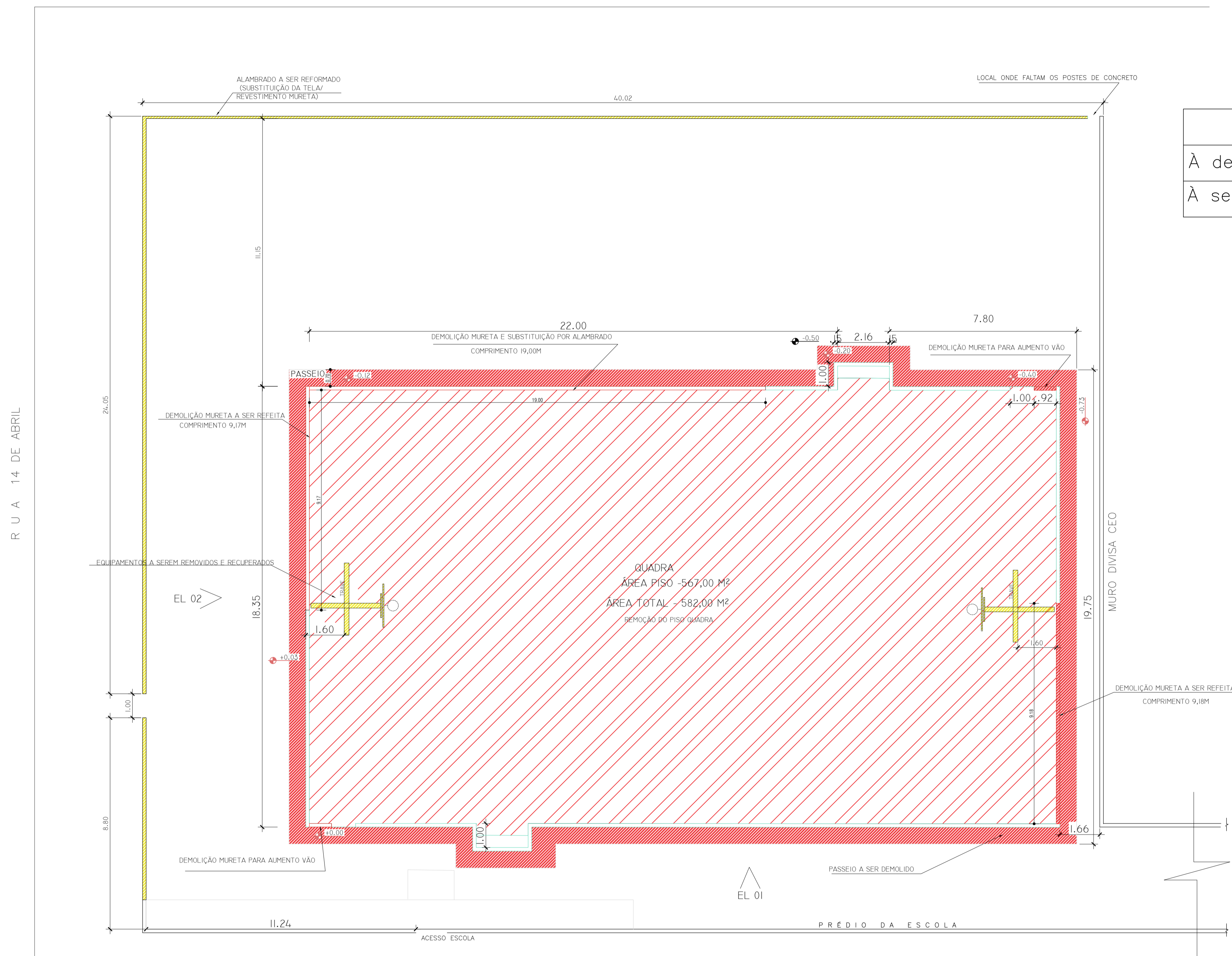
PLANTA BAIXA – demolição/remoção ESC: 1/100
