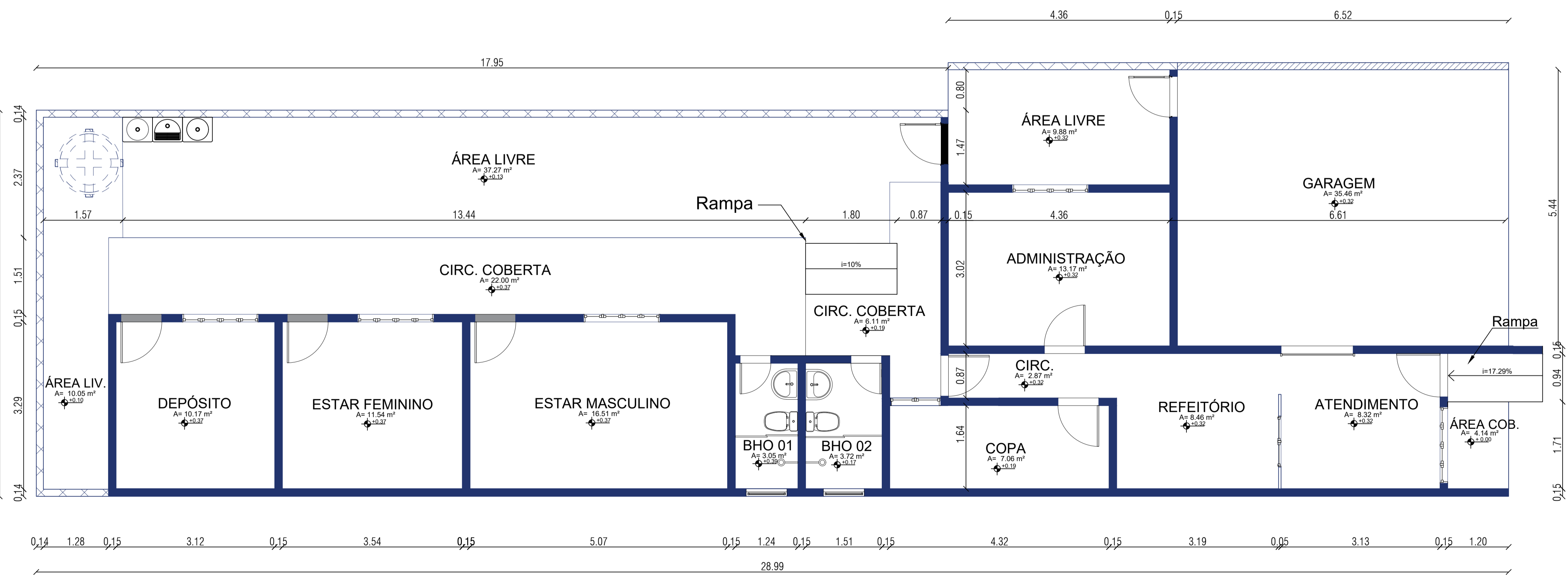
02 PLANTA BAIXA - PROPOSTA ESC. 1/50
