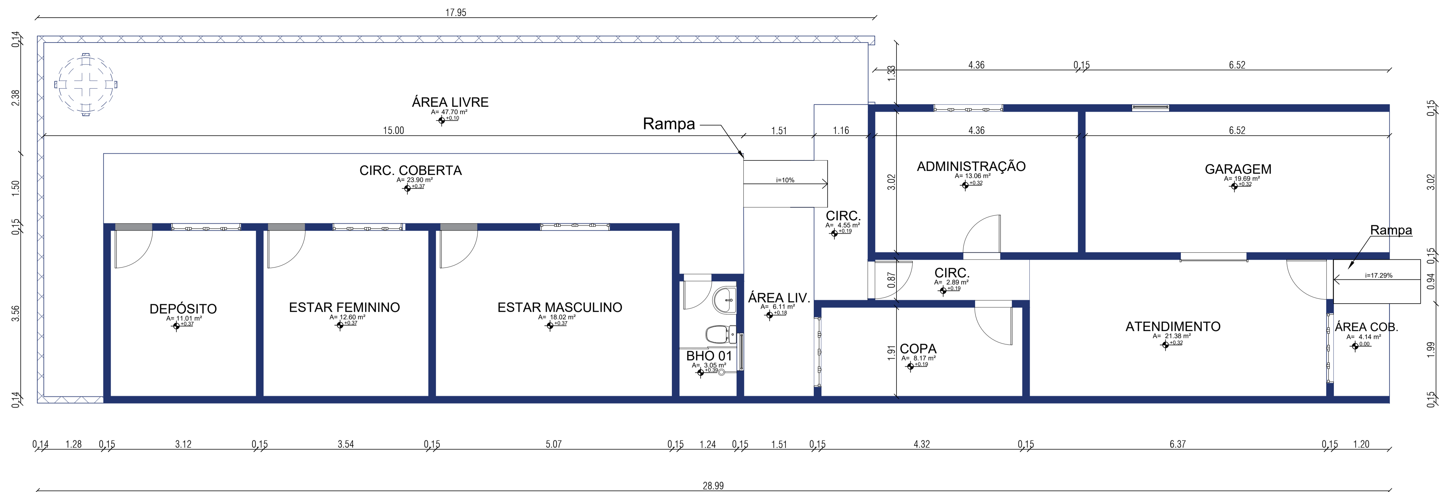
01 PLANTA BAIXA - ATUAL ESC. 1/50
