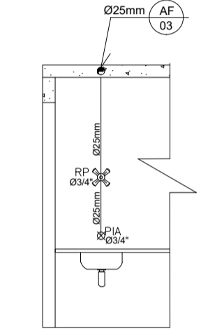
DETALHE H3
