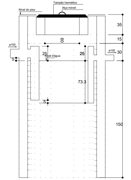
TANQUE SÉPTICO CORTE - ESC. 1:25
