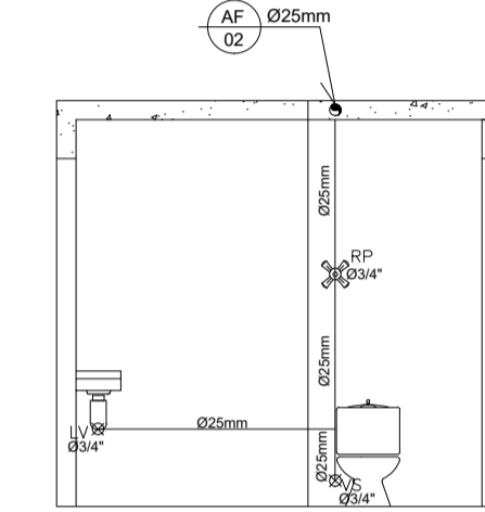
DETALHE H2
