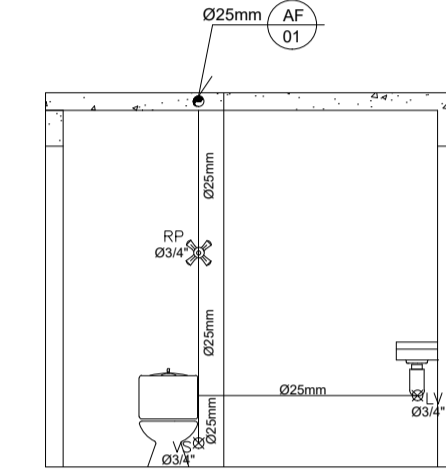
DETALHE H1
