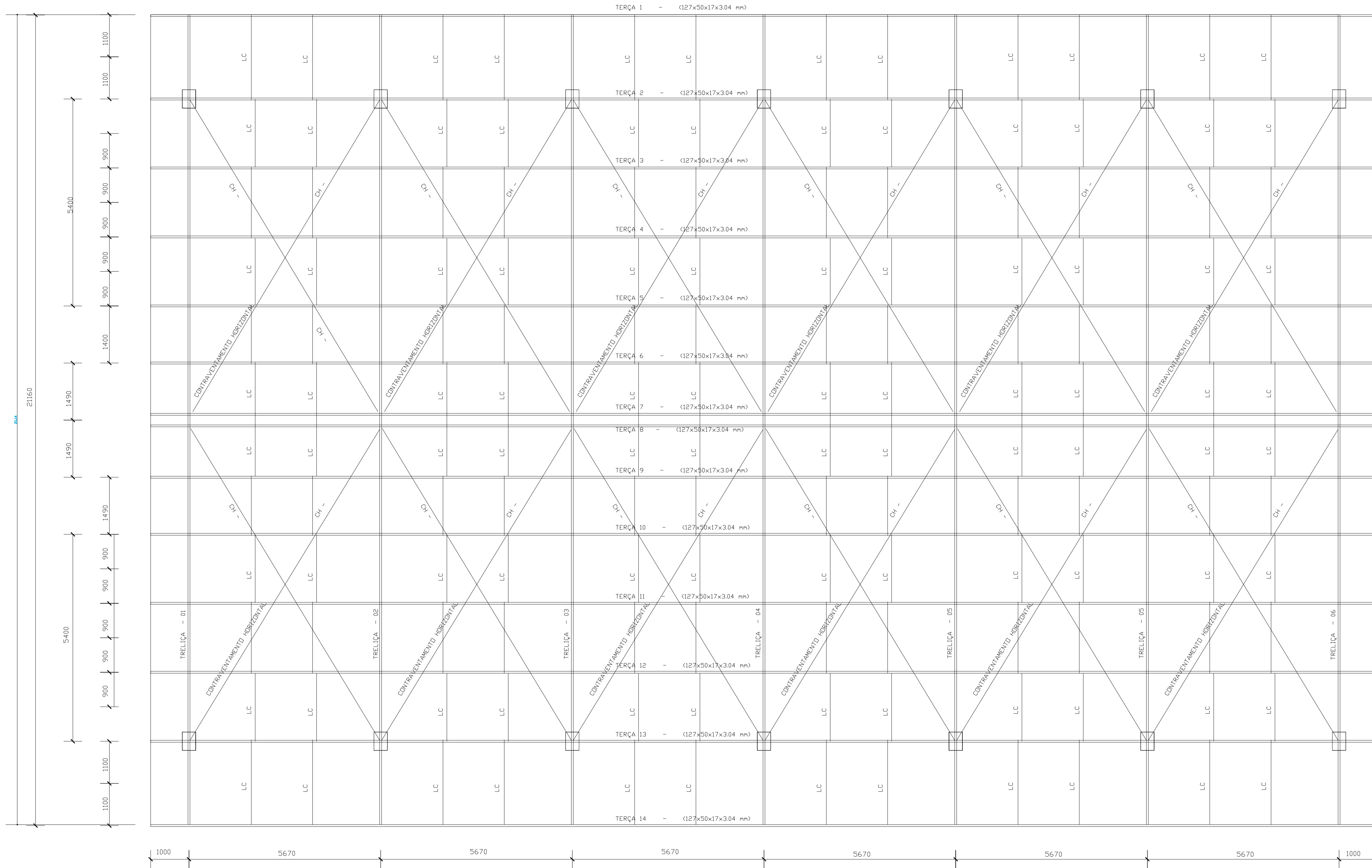
IMPLANTAÇÃO DA COBERTURA ESC: 1/50
